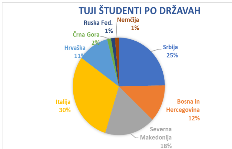
Graf 2: Število vpisanih tujih študentov po državah
